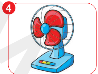
afn fan
