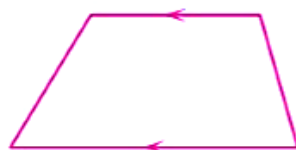
شبه منحرف
