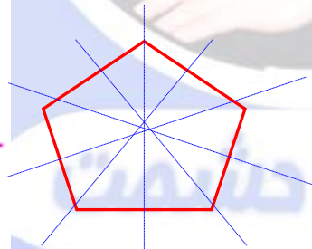
خماسي منتظم
